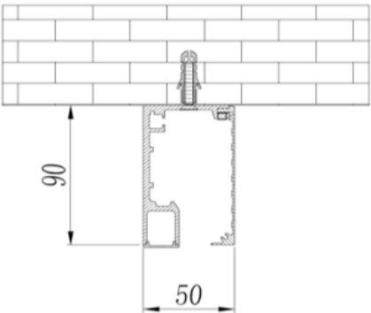
PERFIL DE ALUMINIO
